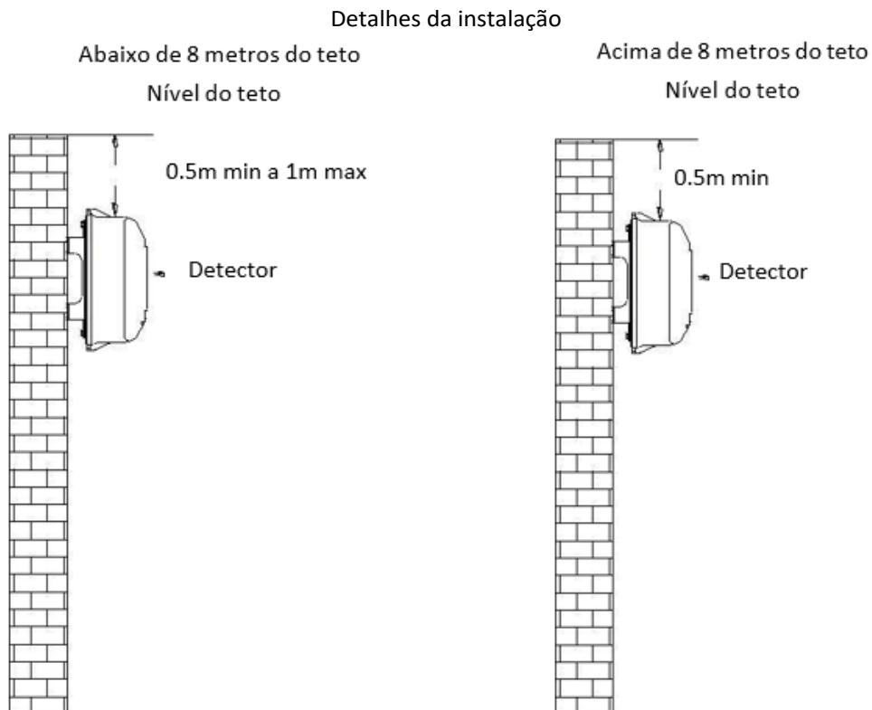
Figura 3: Diagrama de instalação
