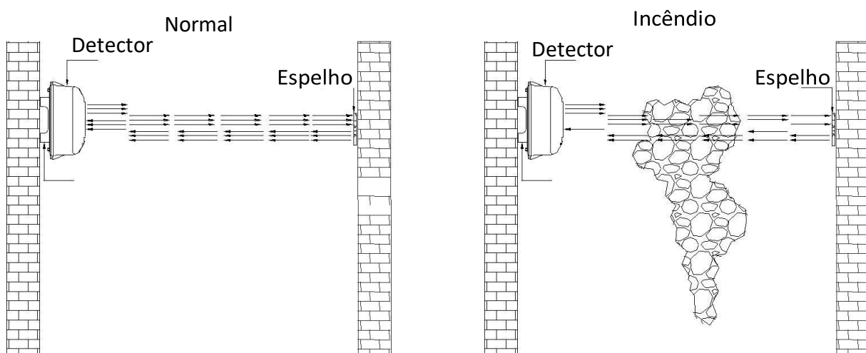
Figura 1: Princípios do Detector
