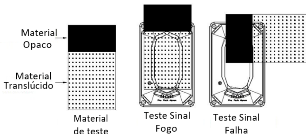
Figura 9: Detalhes de teste
