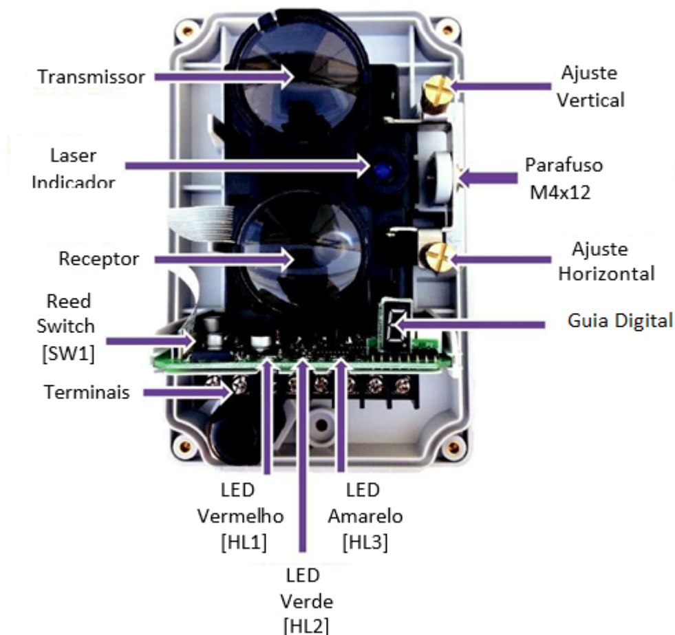
Figura 8: Detalhes do Detector
