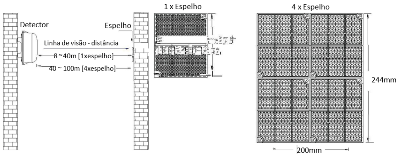
Figura 6: Montagem do espelho
