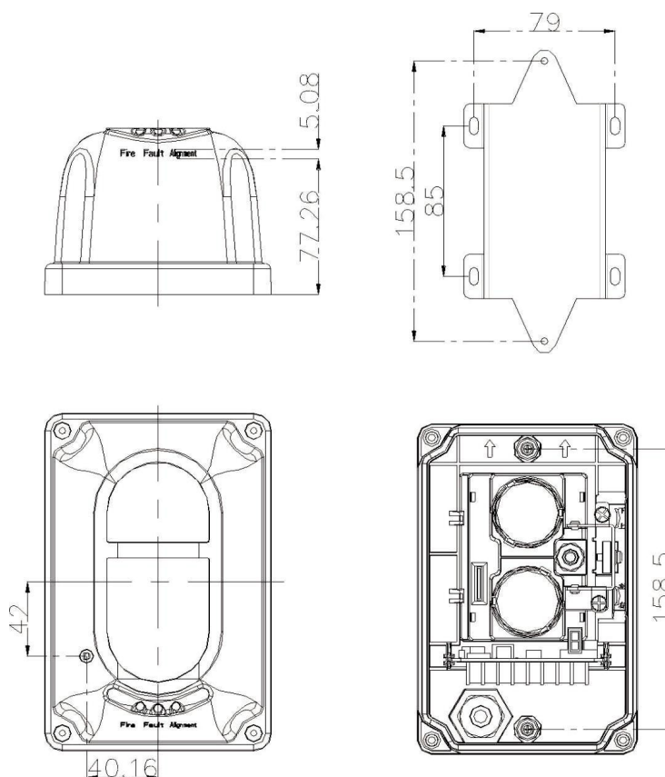
Figura 2: Diagrama do Detector
