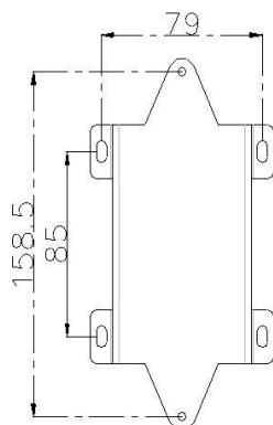
Figure 4: Base de Montagem
