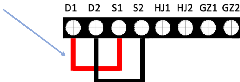
Figura 7: Terminais de fiação
